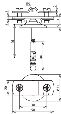
Maßbild
