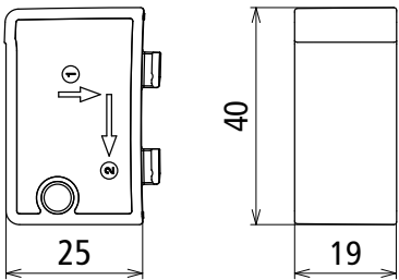
Maßbild
