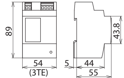
Maßbild
