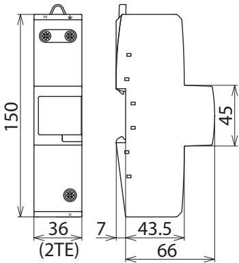
Maßbild DGPM 1 255
