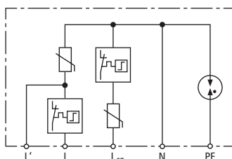
Prinzipschaltbild DCOR L 3P 275 SO IP
