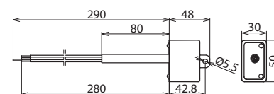
Maßbild DCOR L 3P 275 SO IP
