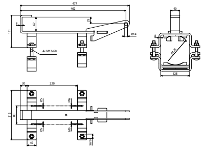
Maßbild HA VH BO GSH 27 VC
