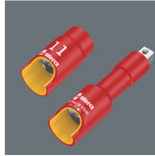
Die Zyklus Nüsse und -Verlängerungen für Elektriker bieten eine erhöhte Sicherheit durch ihre 2-komponentige Isolation mit gelbem Isolationskern unter roter Isolationsaußenschicht.
