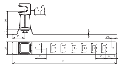
Maßbild DLH US 8 H36 L205 GR V2A
