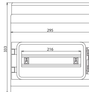
Maßbild IGA 12 IP54
