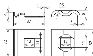
Maßbild KP AQ4 50 DUL 8.10 VKL11 V2A
