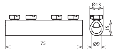
Maßbild VM 8 SKM6X8 CU
