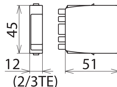
Maßbild BXT ML2 BD S 12
