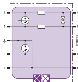
Prinzipschaltbild BXT ML2 BD S 12
