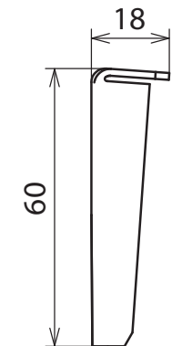
Maßbild KEIL BES NIRO
