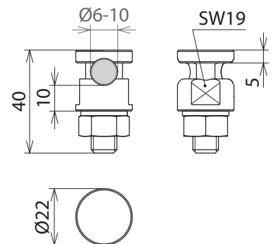
Maßbild UKSV 6.10 AQ16 50 V4A
