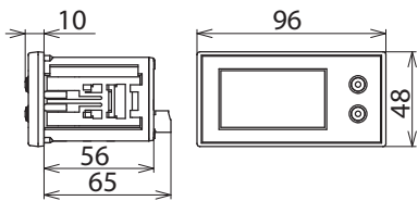
Maßbild DPAN L
