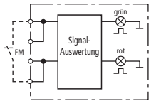
Prinzipschaltbild DPAN L
