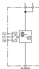
Prinzipschaltbild DBM 1 440 FM
