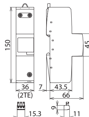
Maßbild DBM 1 440 FM
