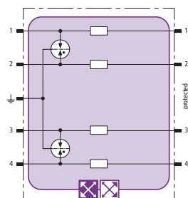
Prinzipschaltbild BXT ML4 B 180
