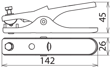
Maßbild EZ 16 FL13 ASM6 STGALZN
