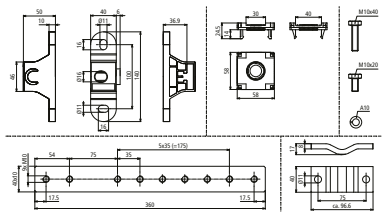
Maßbild PAS EX 1+5AP M10 V2A
