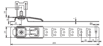
Maßbild DLH UG 8 H20 L205 KT V2A
