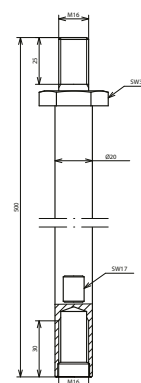
Maßbild TE 20 500 M16 STTZN
