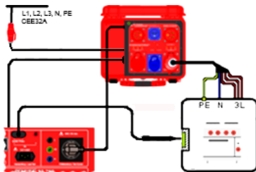
Anschlussschema
