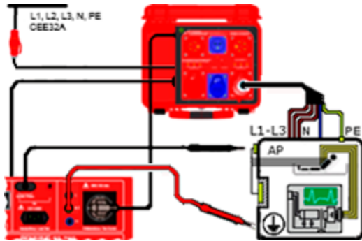
Anschlussschema
