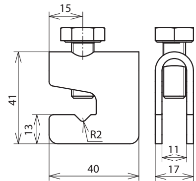
Maßbild VK A UNI ST
