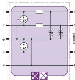
Prinzipschaltbild BXT ML2 BE S 36
