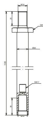
Maßbild TE 20 1500 M16 STTZN
