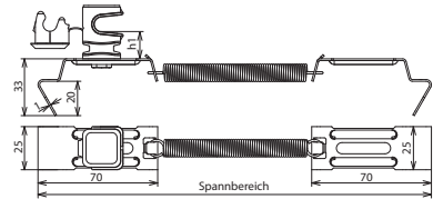
Maßbild DLH SS 8 H16 FG180.280 GR V2A
