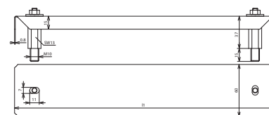
Maßbild AD PAS 6AP V2A
