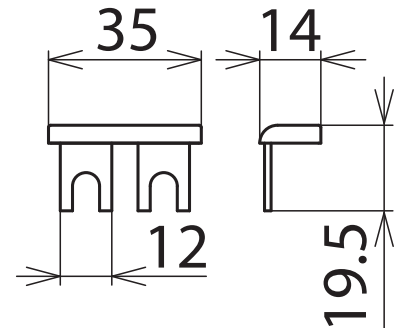
Maßbild MVS 1 2
