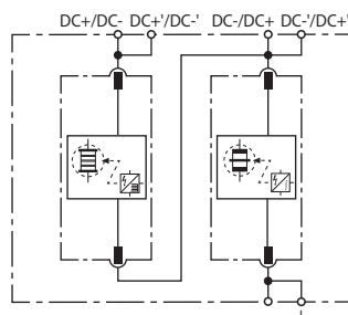
Prinzipialschaltbild DSE M 2P 60
