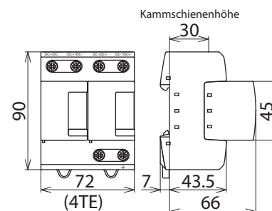
Maßbild DSE M 2P 60
