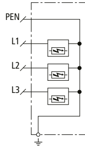
Prinzipschaltbild
