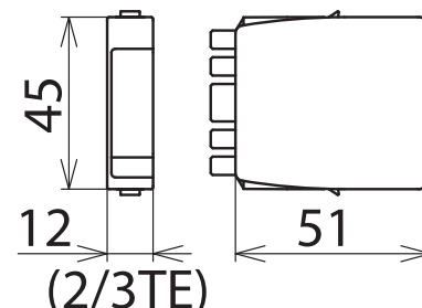
Maßbild BXT ML2 BE S 12
