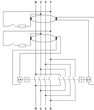
Anschlussschema
