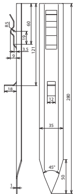
Maßbild AH FE RF
