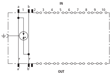
Prinzipschaltbild DRL 10 B 180
