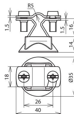
Maßbild LH ZS 8.10 FL20 M8 KS V2A
