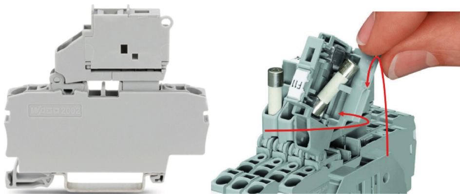
Abbildung 18. Austauschen der Feinsicherungen
