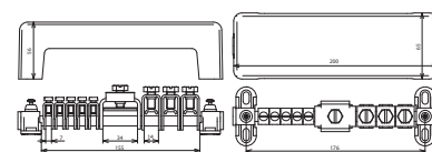
Maßbild PAS AH RK 5X25 3X8.10 1XFL30
