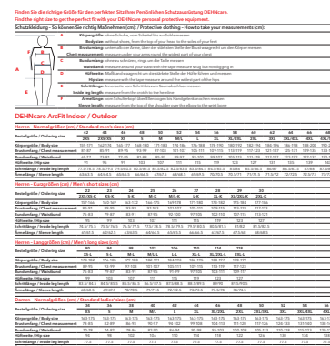
Maßbild APT OD YE 58
