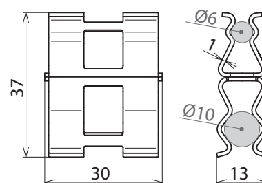
Maßbild DC BK 6 RD10 STBLANK
