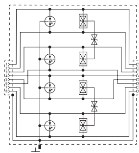
Prinzipschaltbild DPA CLE IP66
