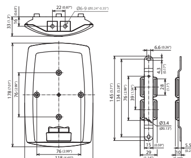
Maßbild DPA CLE IP66
