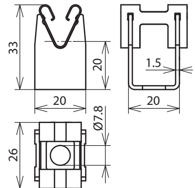
Maßbild LH DG 8 H20 B7.8 CU
