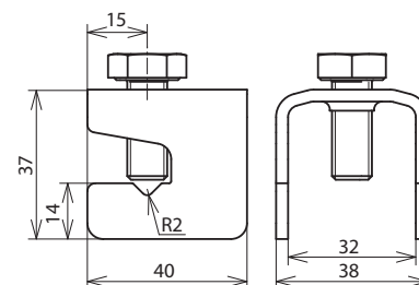
Maßbild VK 6.10 FL30 FL30 BSB STTZN
