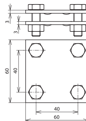
Maßbild KS FL30 V4A
