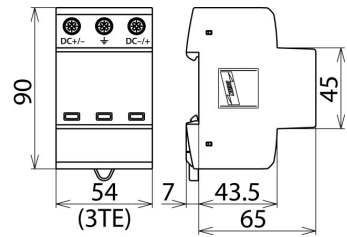
Maßbild DG YPV SCI 1000
