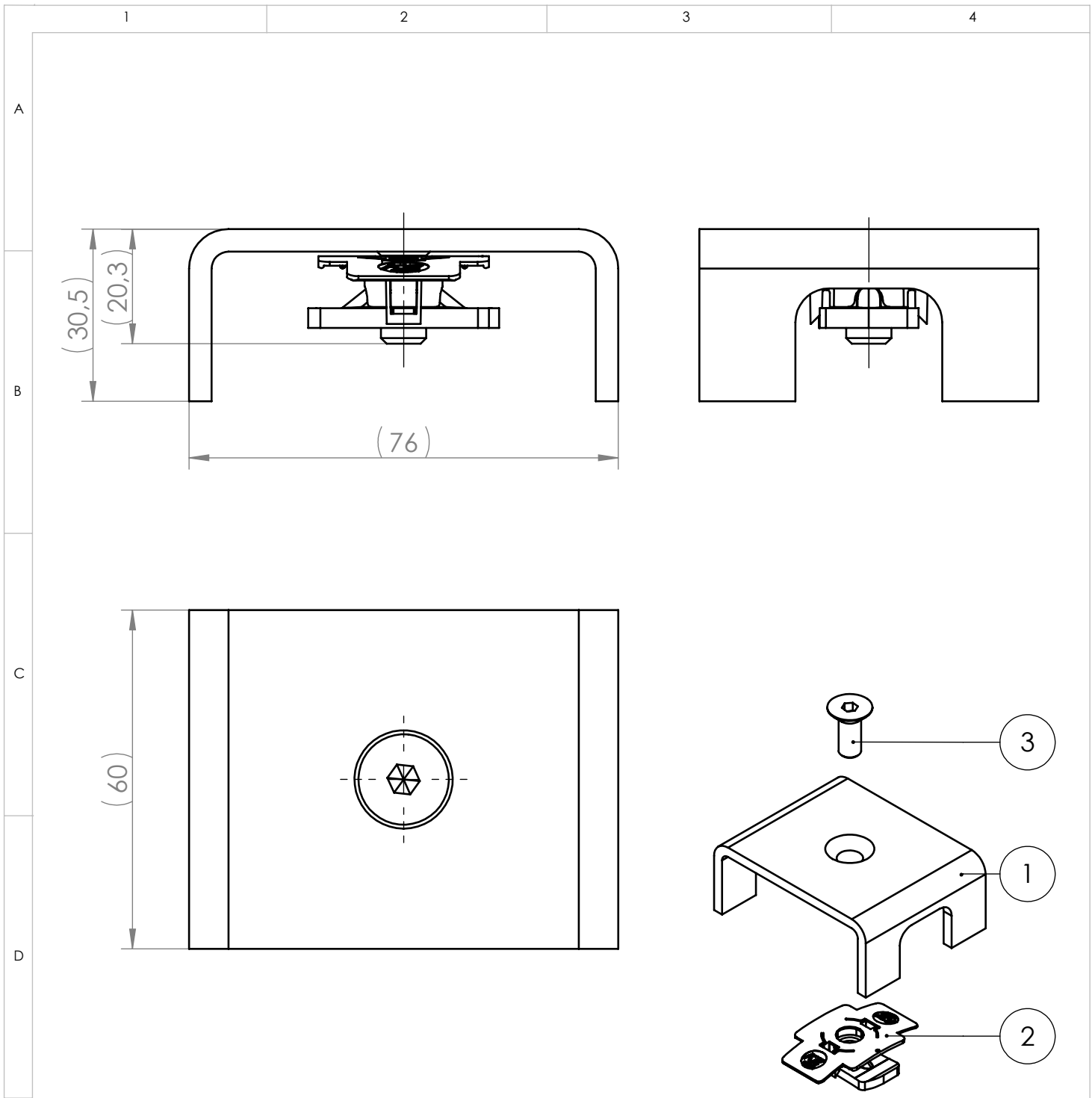
Isometrie 1:2
