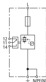
Prinzipialschaltbild DBM 1 CI 440 FM
