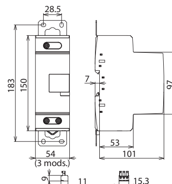
Maßbild DBM 1 CI 440 FM
