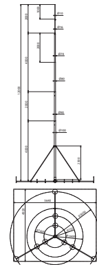
Maßbild FS D100 10 12M AL DBS STTZN
