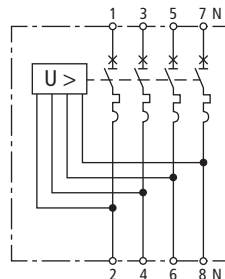
Prinzipschaltbild POP 4 255 C25
