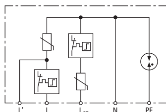
Prinzipschaltbild DCOR L 3P 275 SO LTG
