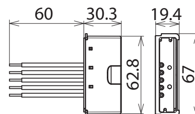
Maßbild DCOR L 3P 275 SO LTG
