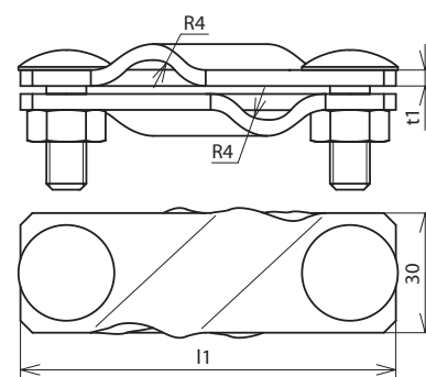
Maßbild SVK 7.10 7.10 FL30 STTZN
